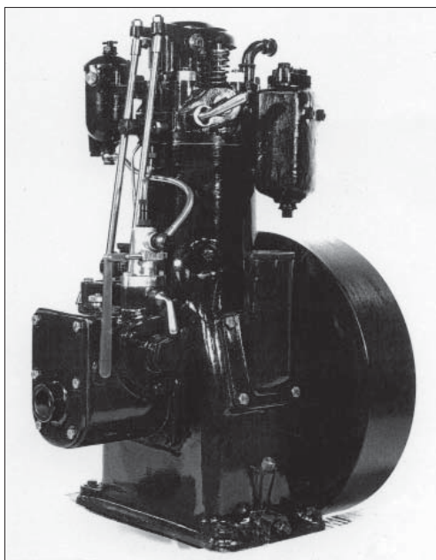
Motor Josman. Foto cedida per Manuel Font Canós
