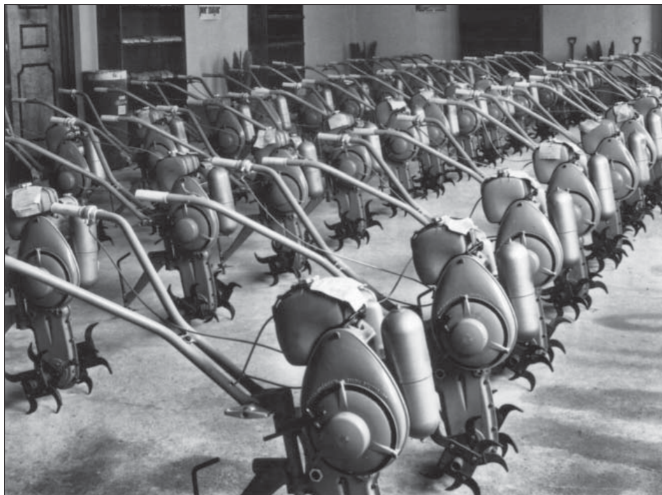
Solo model Minor, en l'exposició de Metalúrgica Santa Helena ©Arxiu Flores-Llorens
