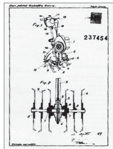
Expedient de patent del motocultor Solo ©Arxiu de Patents i Marques
