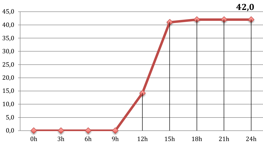
Evolución lluvia acumulada en VILA-REAL el 02/09/23 (en l/m 2 )
