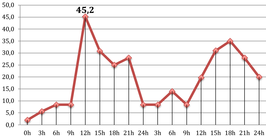
Ráfagas de viento máximas en periodos de 3 horas, registradas en VILA-REAL el 02 y 03/09/23 (en km/h)
